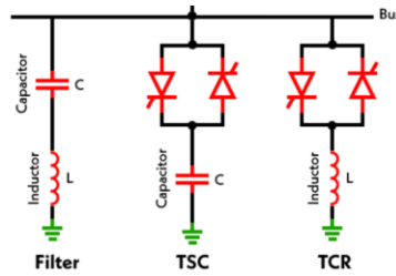
Fig. 5: Construction of SVC [28].
